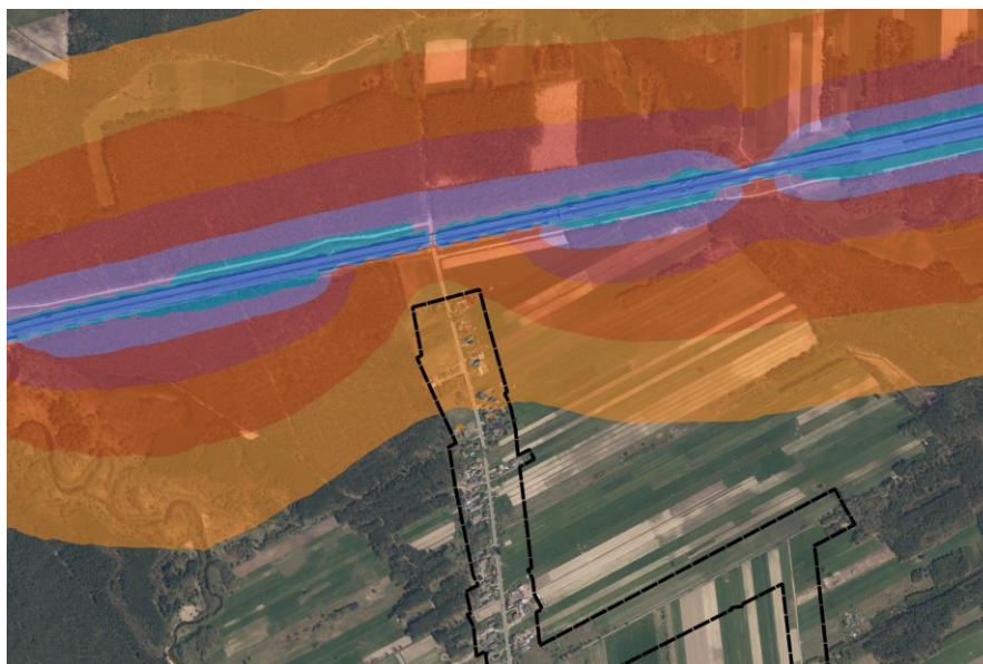
Mapa imisyjna dla wskaźnika L_{DWN} w rejonie obrębu Ldzań
