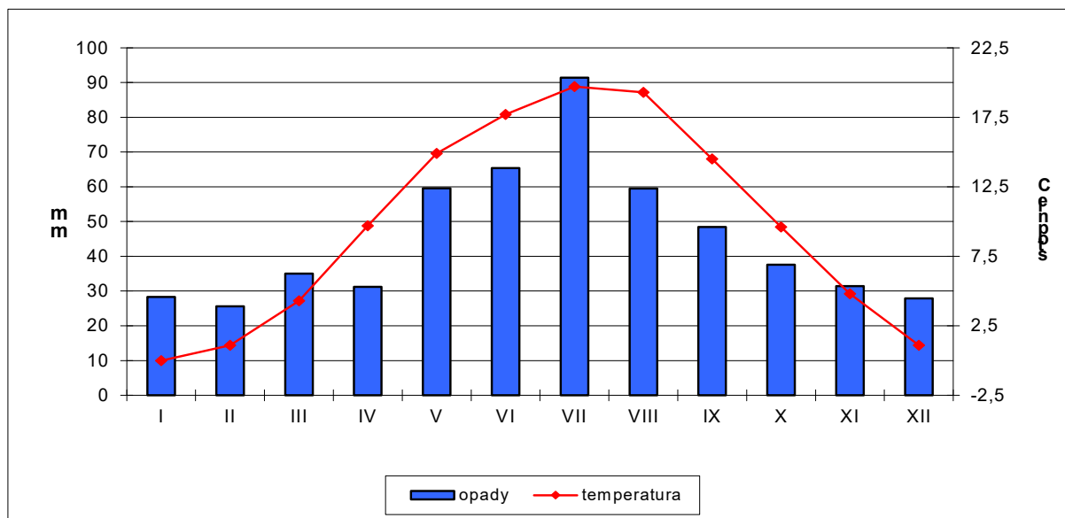
RYCINA 1: Rozkład średnich temperatur oraz sum opadów dla Wrocławia w latach 1991 – 2020.
