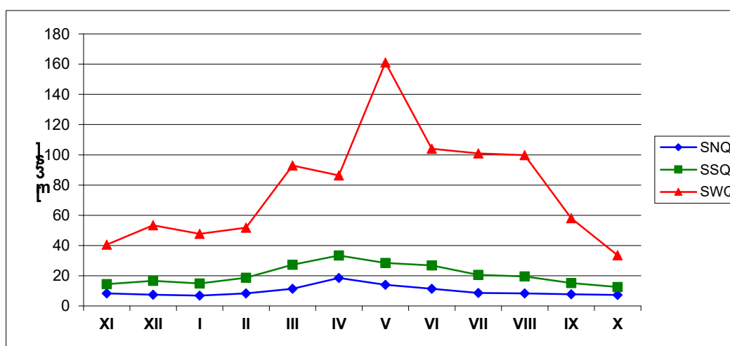
RYCINA 4: Charakterystyczne przepływy wody rzeki Nysy Kłodzkiej (m³/s) w okresie 1959 – 1974 na profilu Byczeń.
