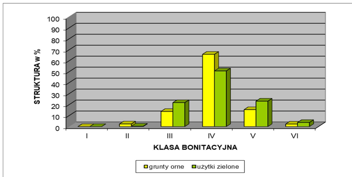
RYCINA 5: Struktura powierzchni gruntów ornych i użytków zielonych według klas bonitacyjnych 17 .
