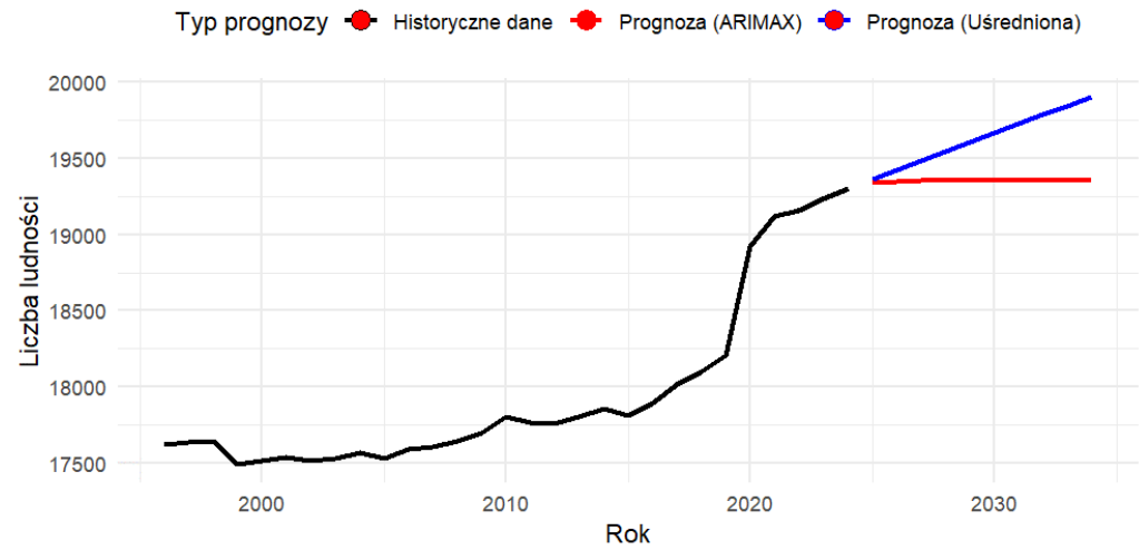
Porównanie prognozy uśrednionej i ARIMAX
