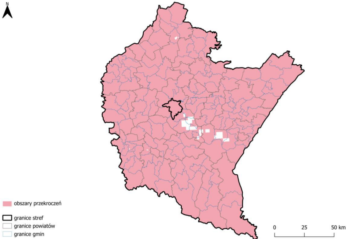
Rysunek 18 Zasięg obszarów przekroczeń poziomu docelowego ozonu dla 8-godz. stężenia O_3 ze względu na ochronę zdrowia w województwie podkarpackim w 2024 r. [źródło: GIOŚ]
