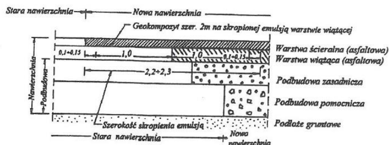
Rys. 2. Konstrukcja połączenia starej i nowej nawierzchni
