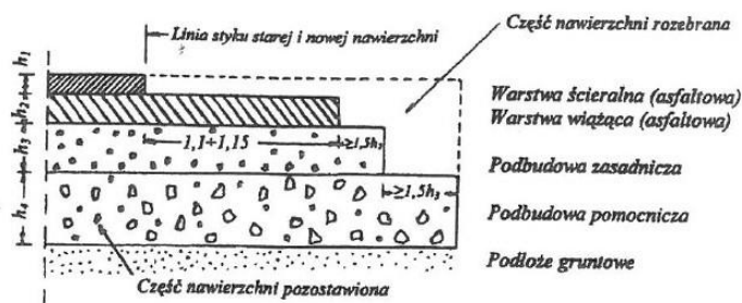
Rys. 2. Konstrukcja połączenia starej i nowej nawierzchni
